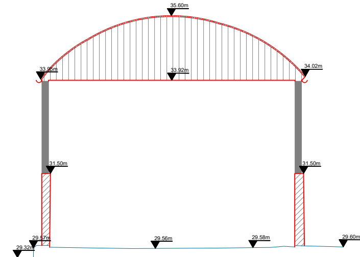
ELEVATION 1
