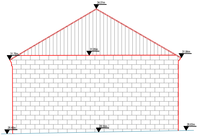
ELEVATION 2
