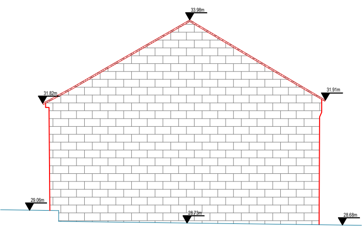
ELEVATION 4
