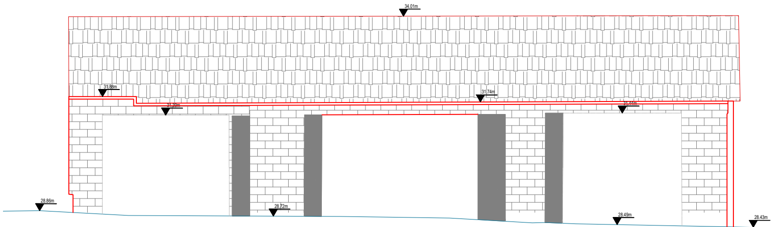
ELEVATION 1
